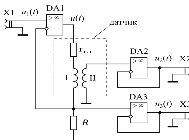
Рисунок 1. Принципиальная схема выносного блока учебного лабораторного комплекса.
